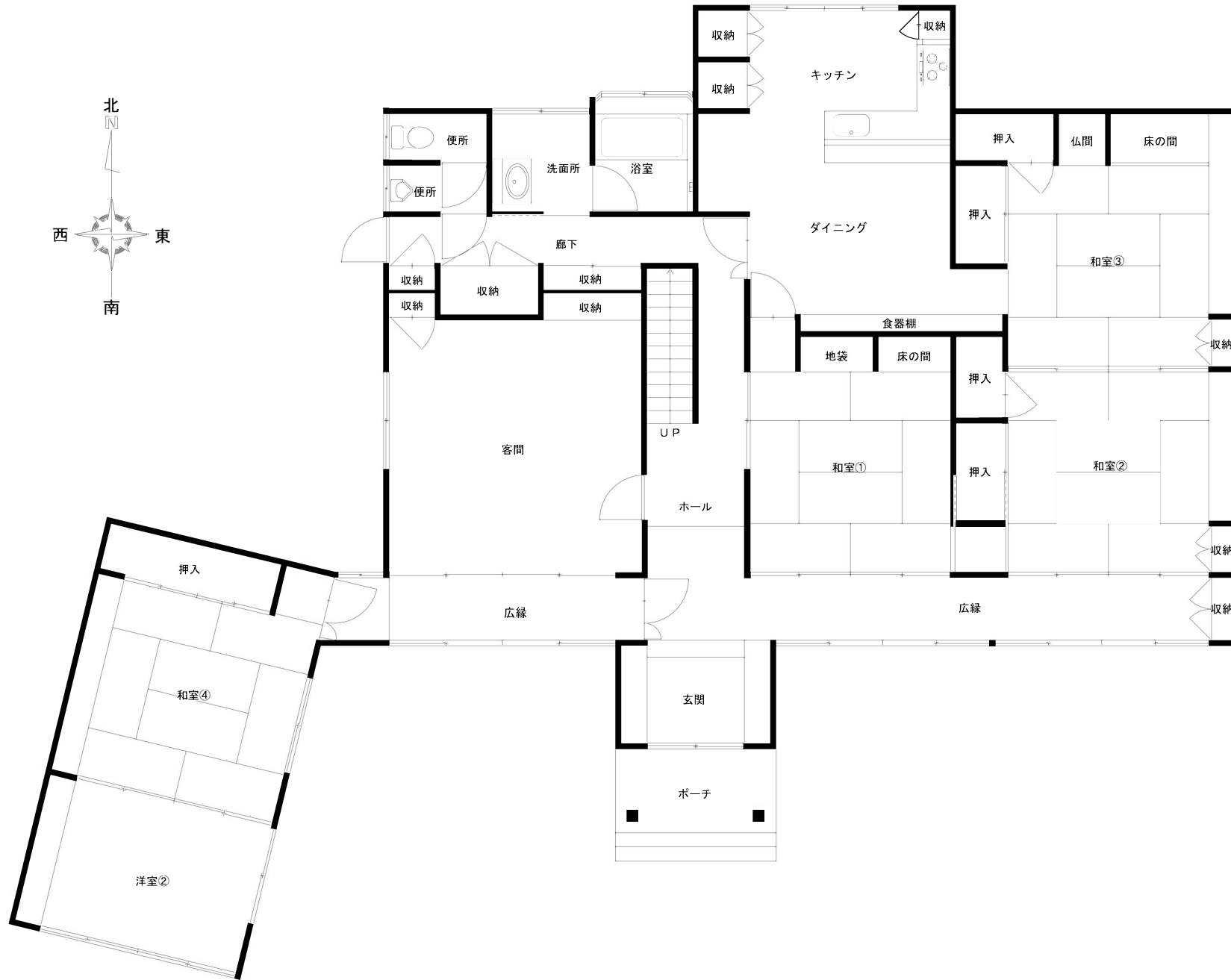
1階平面図
