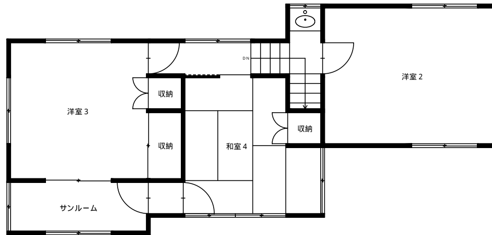
2 階平面図
