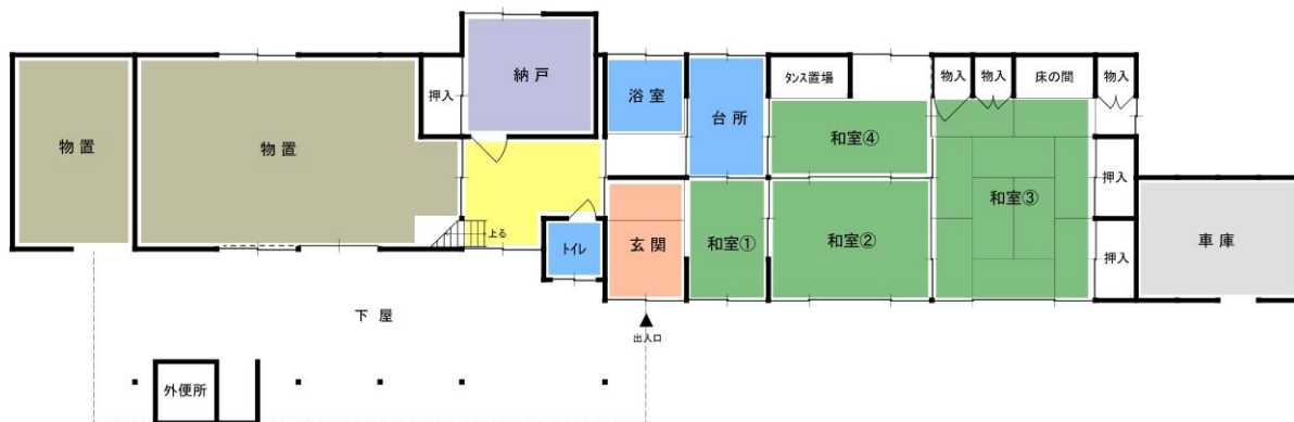
1階平面図
