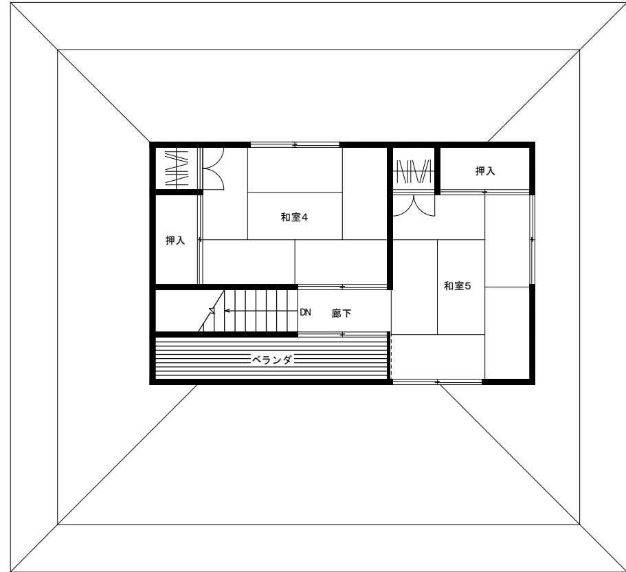
2階平面図
