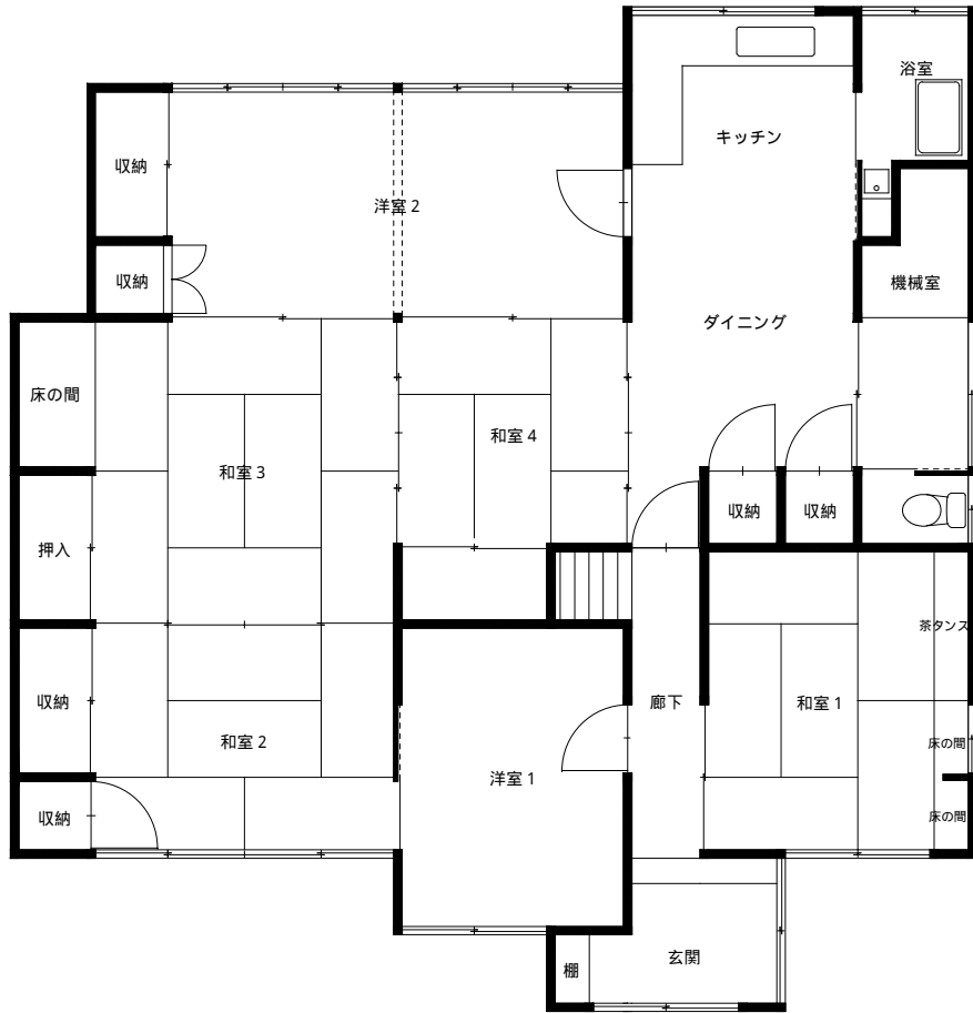
1階平面図
